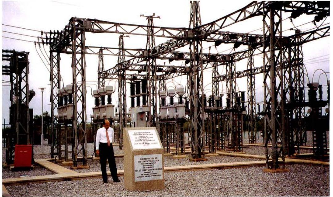
ガーナ国 ソガコーベ変電所
