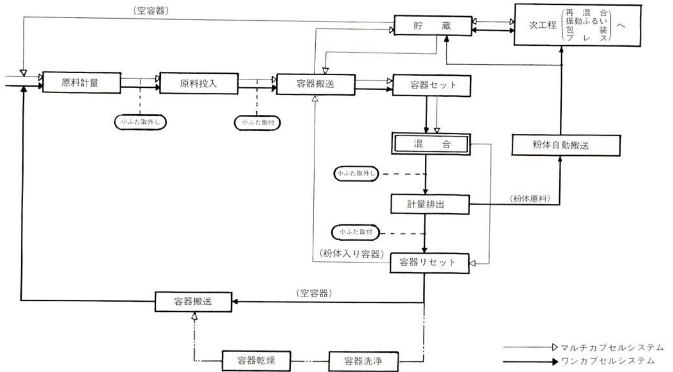
図9(b)/自動混合システムフロー Fig. 9 b)/ Flow diagram of automatic mixing system
